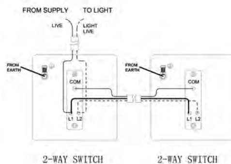
2 WAY SWITCH
